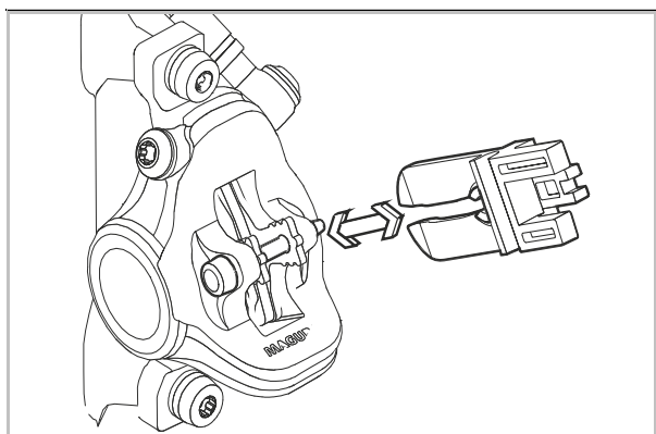
Illustration 65 : Insérer la cale de transport
