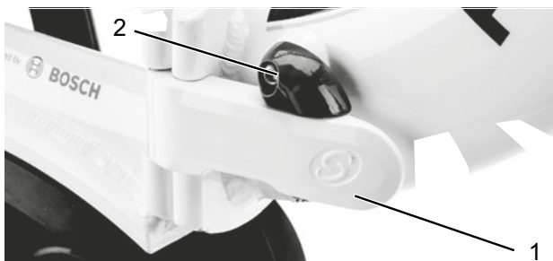
Illustration 140 : Levier de serrage du cadre fermé (1) et levier de blocage du cadre fermé (2)
