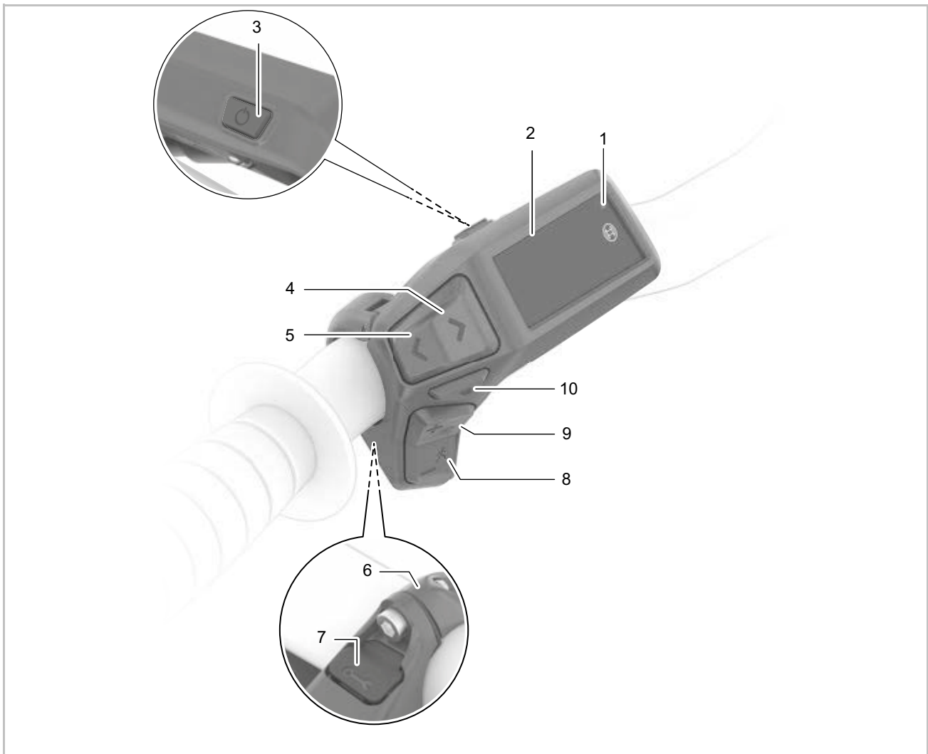
Illustration 53 : Aperçu de l'ordinateur de bord BOSCH LED Remote
