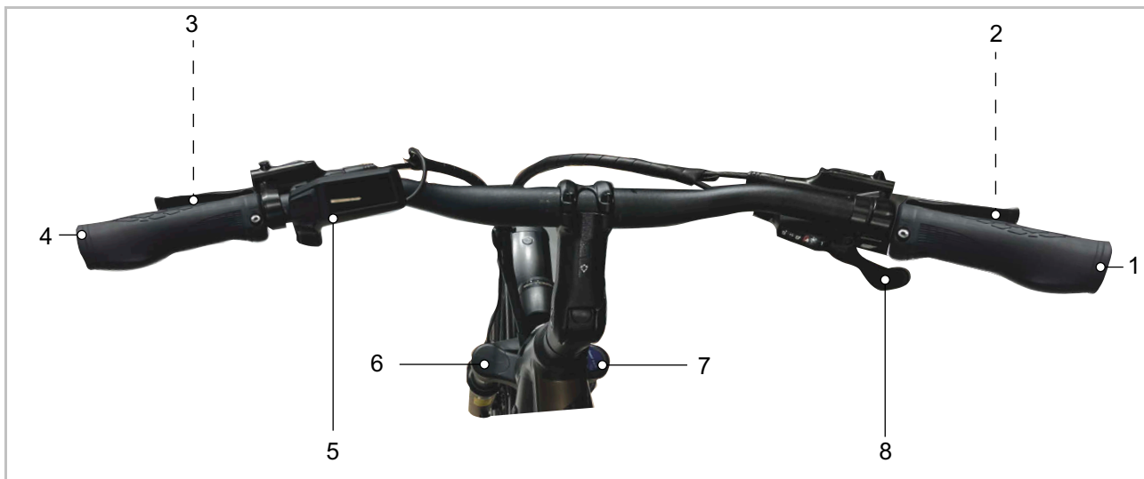
Illustration 52 : Vue détaillée d'un guidon avec BOSCH Purion 200, exemple
