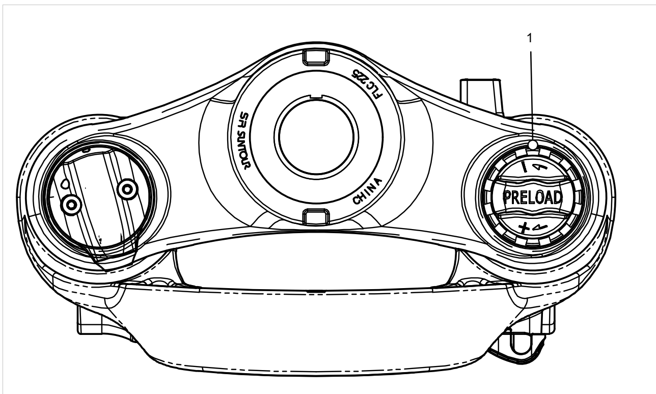
Illustration 123 : Exemple d'une SR SUNTOUR, molette de réglage du sag sur la couronne de fourche
