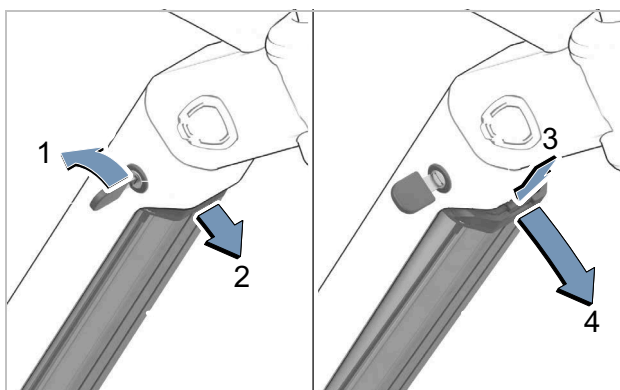
Illustration 143 : Retirer la batterie intégrée
