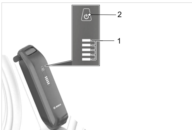
Illustration 57 : Éléments d'affichage et de commande de la batterie BOSCH PowerPack
