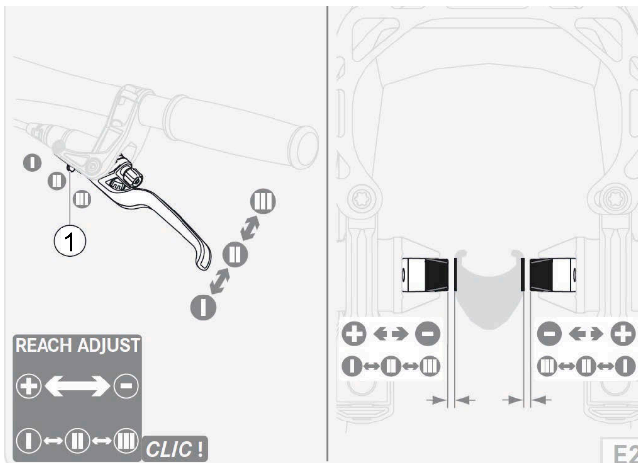
Illustration 117 : Réglage de la garde d'un frein à main MAGURA HS22
