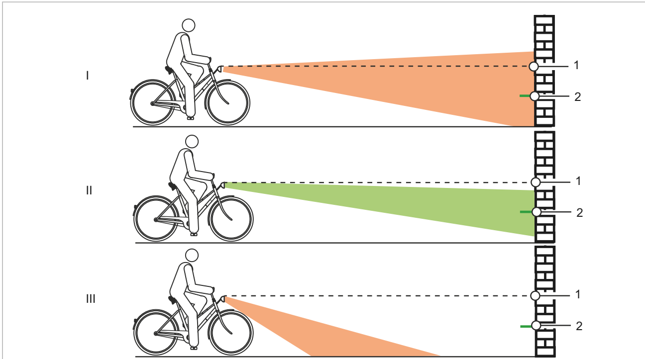
Illustration 194 : Feu réglé trop haut (1), correctement (2) et trop bas (3)
