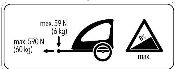
Illustration 138 : Plaque d'information de la remorque
