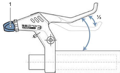
Illustration 183 : Tournez la vis de réglage (1) jusqu'à ce que les freins agissent après \frac{1}{3} de course du frein à main
