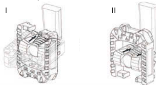
Illustration 168 : Plier la pédale vers le bas (I) ou vers le haut (II)
