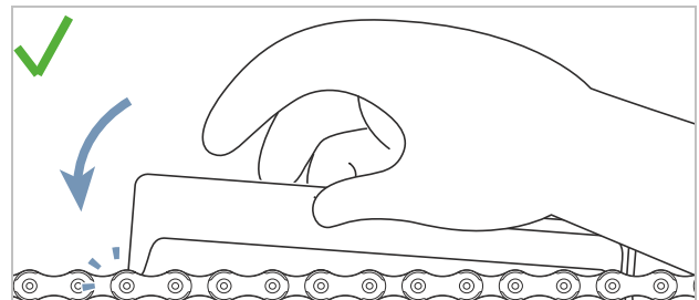
Afbeelding 192: Kaliber past niet
