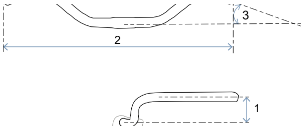
Afbeelding 6: Maten stuur
