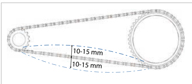
Afbeelding 184: Voorbeeld kettingspanning controleren: 5 mm omhoog, 10 mm omlaag = 15 mm uitwijking
