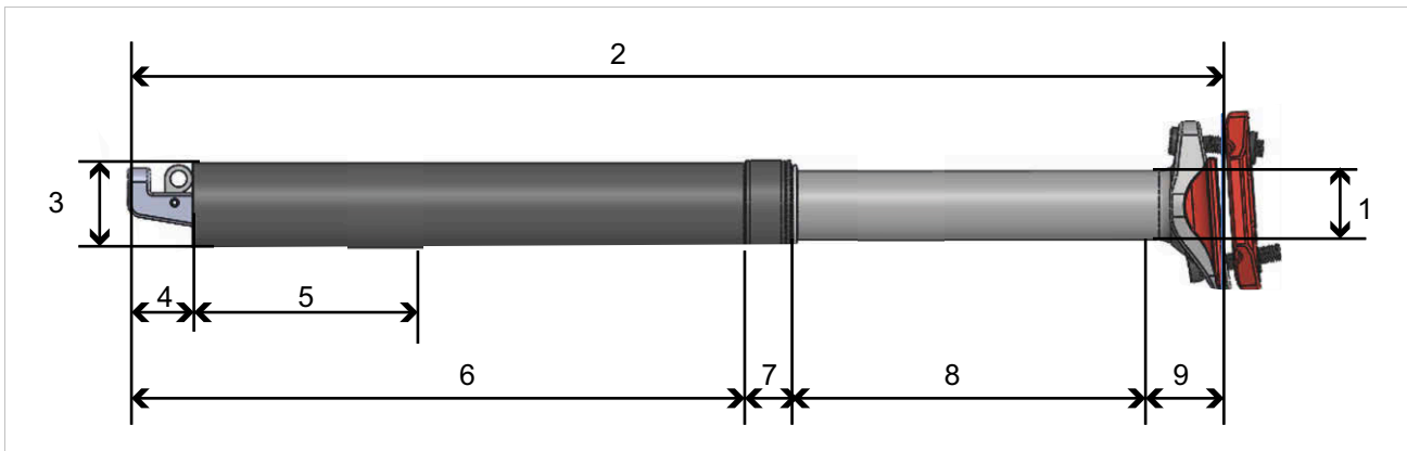
Afbeelding 44: Afmetingen zadelpen LIMOTEC, A1L
