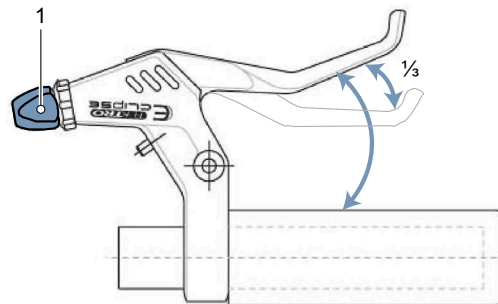
Afbeelding 183: Stelschroef (1) draaien tot het remmen na \frac{1}{3} van de afgelegde weg van de handrem inzet
