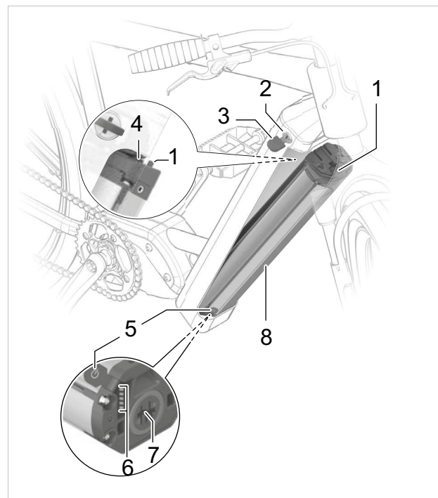
Afbeelding 50: Details PowerTube
