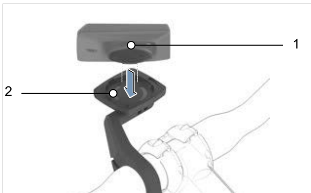
Afbeelding 134: Display aanbrenge
