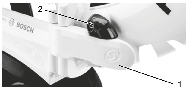
Afbeelding 140: Gesloten framespanhendel (1) en gesloten framevergrendelhendel (2)
