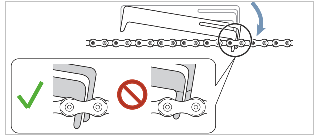
Afbeelding 190: Kaliber wordt ingestoken
