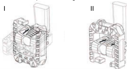
Afbeelding 168: Pedaal omlaag (I) of omhoog (II) invouwen
