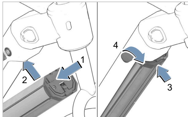
Afbeelding 144: Geïntegreerde accu aanbrengen
