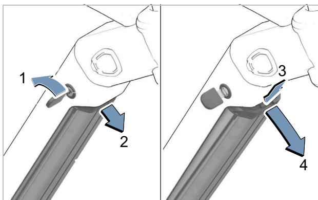
Afbeelding 143: Geïntegreerde accu verwijderen
